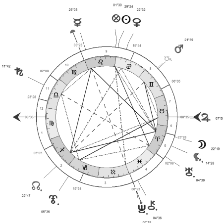
Fig 1 : l'horoscope de l'attentat d'Oslo
