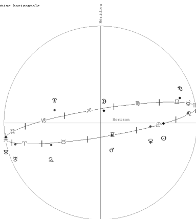
Fig. 3 : perspective horizontale montrant à quel point l'écliptique est couchée sur l'horizon. La Lune, bien que proche du méridien, a une hauteur très faible.
