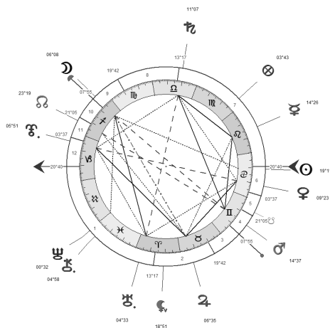
Fig.2 : Horoscope pour la première visibilité de la Lune à Oslo le 11 juillet 2011 au coucher du Soleil (20h24 TU). Vue en perspective horizontale. La Lune, au méridien, n'est qu'à environ 7° de hauteur, valeur limite pour être visible. Ceci explique pourquoi, à cette latitude géographique, elle ne peut pas être visible dans une phase antérieure (à ce moment l'écart angulaire Soleil-Lune est pourtant de 137°)
